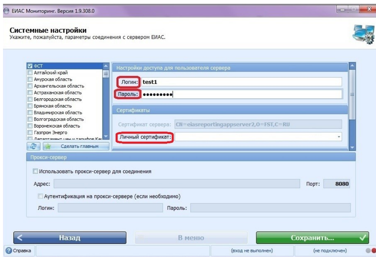
Рисунок 16. Настройка работы с несколькими региональными сегментами
